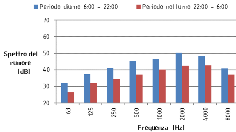
Figura 5 – Spettro del livello globale diurno e notturno nel punto C1
